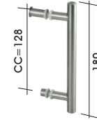
MANILLA + POMO POIGNÉE + BOUTON DOOR PULL + KNOB MANIGLIA + POMOLO *4128/0..
