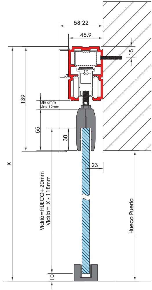
ANCLAJE A PARED
