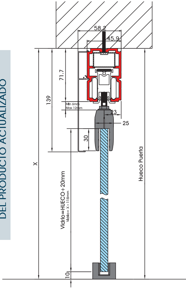
ANCLAJE A TECHO
