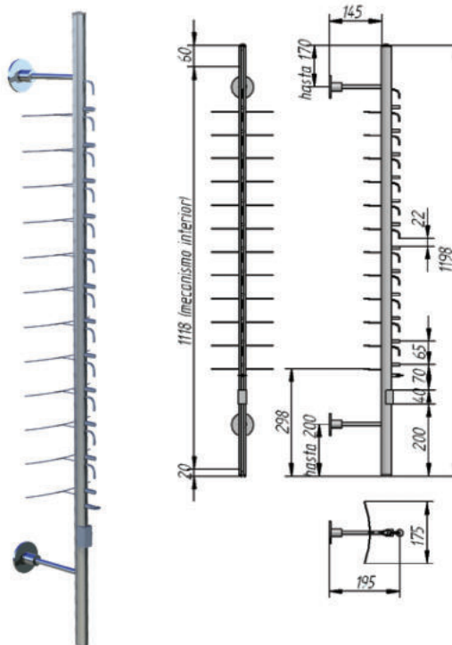
BARRA PARED CON CERRADURA 120 cm 12 gafas - distancia gafas 70 mm
