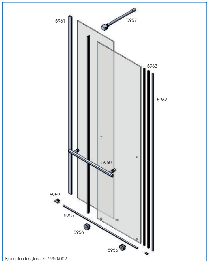
Ejemplo desglose kit 5950/002
