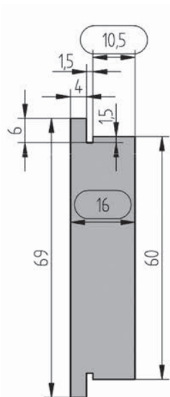
Madera 16 mm
