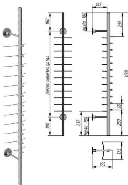
BARRA PARED SIN CERRADURA 120 cm 12 gafas - distancia gafas 65 mm
