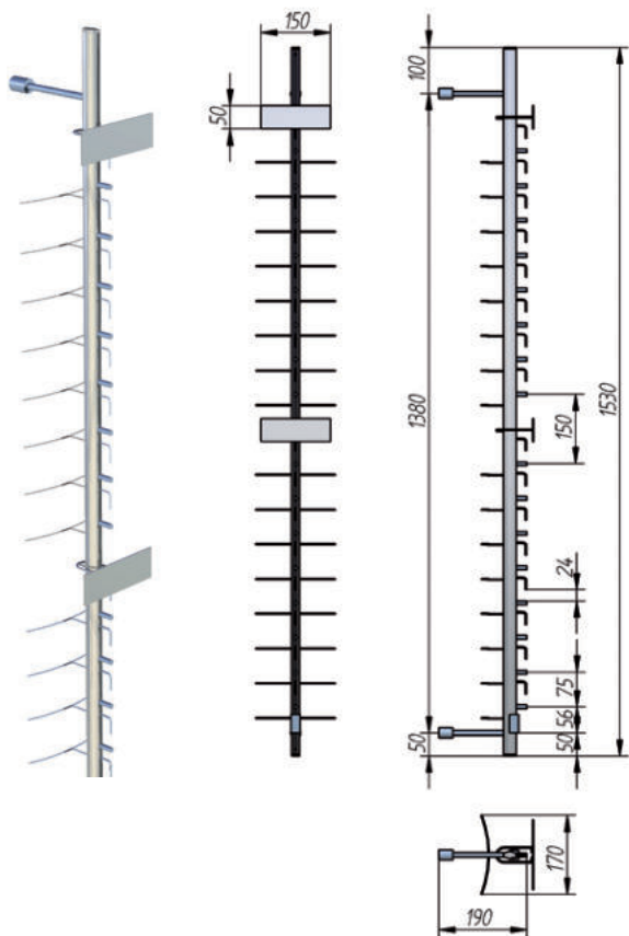
BARRA PARED 8+8 CON CERRADURA 16 gafas - distancia gafas 75 mm
