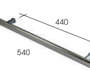
TIRADOR TOALLERO BARRA RECTANGULAR MANILLA + TOALLERO POIGNÉE + SERVIETTE HANDLE WITH TOWEL BAR MANIGLIONE CON PORTA ASCIUGAMANO 5960/032
