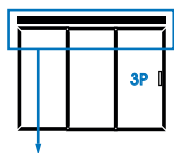
SET COJINETES PARA 3 PUERTAS TELESCÓPICAS JEU DE ROULEMENTS POUR 3 PORTES TÉLESCOPIQUES SET OF FITTINGS FOR 3 TELESCOPIC DOORS SET CUSCINETTI PER 3 ANTE TELESCOPICHE 5201/00N SELF-CLOSING
